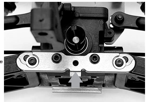
67380 Pivot Plate (RF/3deg) - 7075
